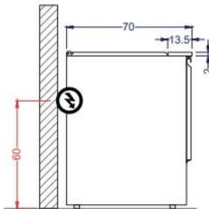
Vista Izquierda
