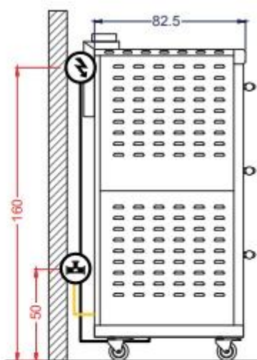
Vista Izquierda
