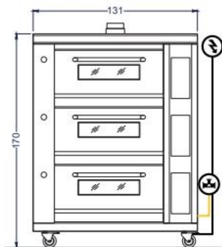
Vista Elevación
